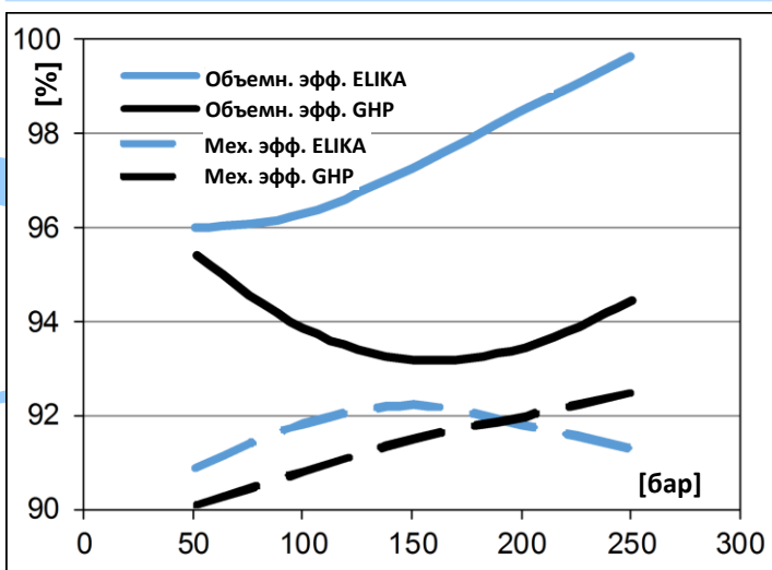
Сравнение эффективности насосов [%]* Marzocchi GHP2 — ELIKA ELI 2: объем одинаковый — 17,8 см 3 /об, скорость вращения 1500 об/мин.
