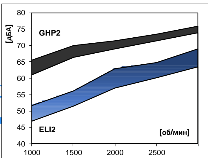
Сравнение уровня шума насосов [дБА]* Marzocchi GHP2 — ELIKA ELI 2: объем одинаковый — 17,8 см 3 /об, давление от 10 до 250 бар.
