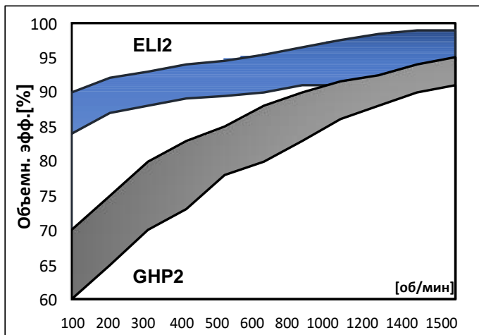
Сравнение объемной эффективности при низкой скорости вращения*: Marzocchi GHP 2 — ELIKA ELI 2, объем 17,8 см 3 /об; P = 200 бар.
