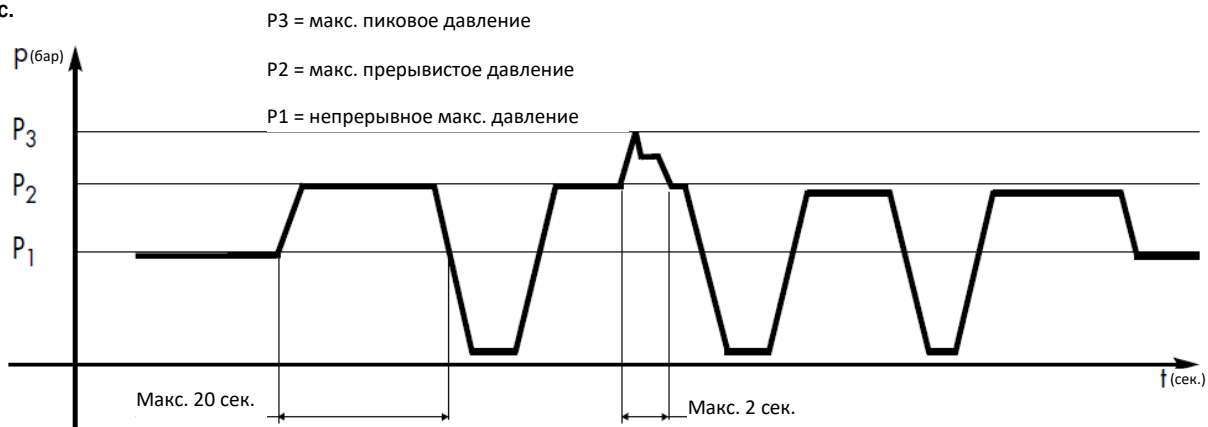
Диаграмма давления как функции от времени.
